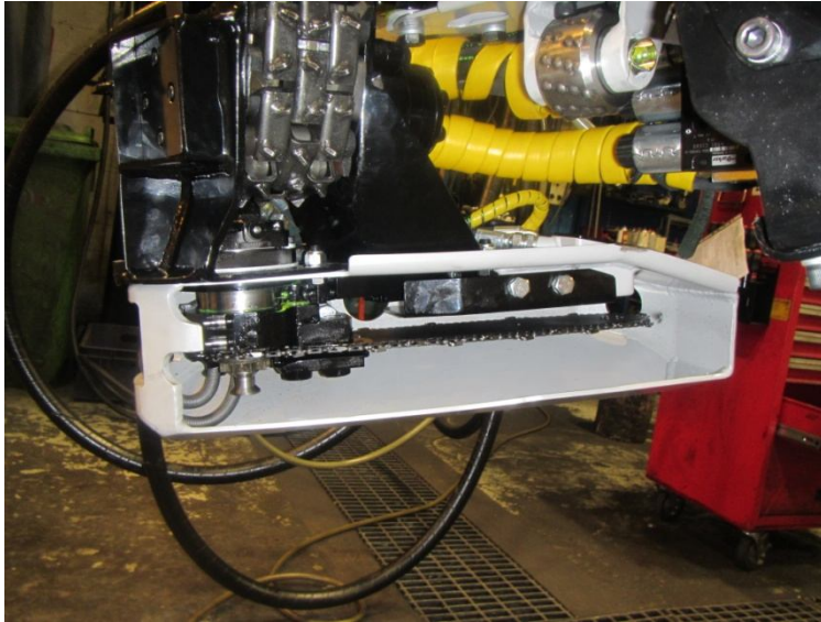
KUVIO 4. Katkaisulaite
