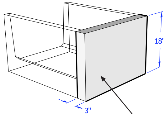
Example: WM2618-03
