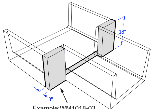
Example: WM1018-03
