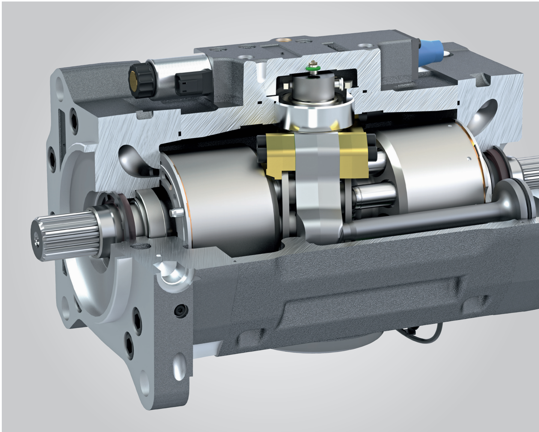
Doppel-Verstellmotor HMV 105-02 D | 210 cm 3 /U | 2 Triebwerke mit gemeinsamer Verstellung und Durchtrieb
