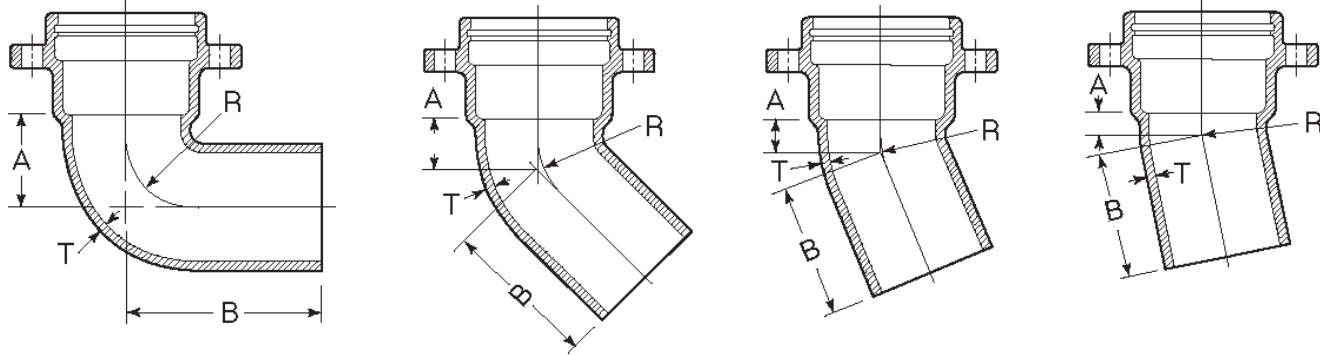
90° (1/4) UT x PE Bends
