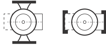
شكل 1 التوجيه الموصى به للصندوق الطرفي
