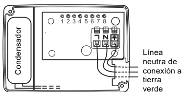
Fig. 3 Diagrama de cableado para todas las bombas de una velocidad (115 V y 230 V)
