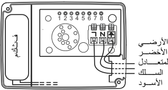
شكل 4 مخطط توصيل الأسلاك للمضخات متعددة السرعات ذات 115 فولت و 230 فولت*
