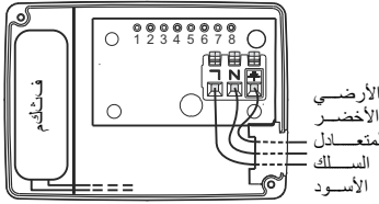
شكل 3 مخطط التوصيل لكل المضخات أحادية السرعة ذات 115 فولت و 230 فولت.
