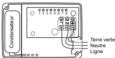
Fig. 3 Schéma de câblage pour toutes les pompes 115 V et 230 V à vitesse unique.
