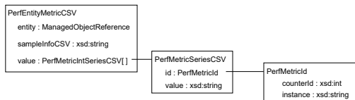
Figure 17-4. PerfEntityMetricCSV Object Hierarchy
