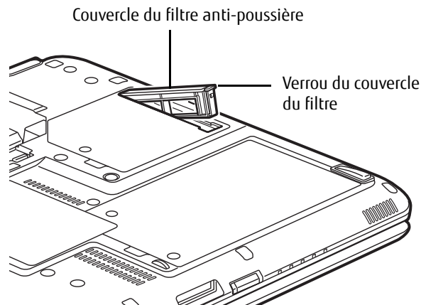
Figure 48. Retrait du couvercle du filtre anti-poussière
