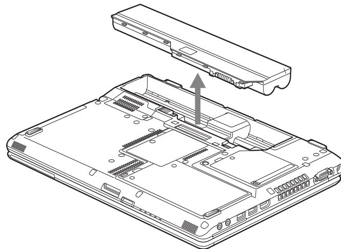
Figure 34. Retrait d'une batterie
