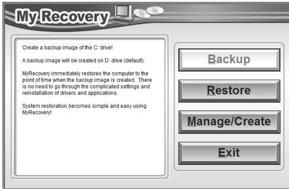
Figure 47. Écran MyRecovery
