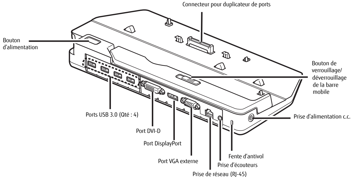
Figure 43. Duplicateur de ports - Arrière
