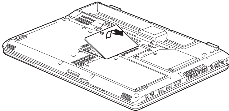
Figure 36. Ouverture du compartiment de mémoire
