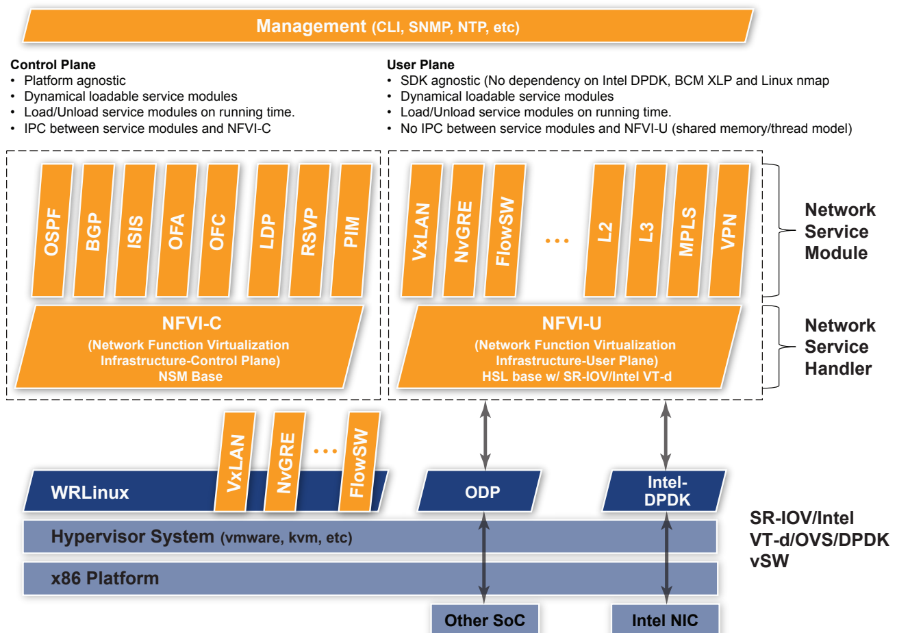
Figure 2. VirNOS: Module Overview
