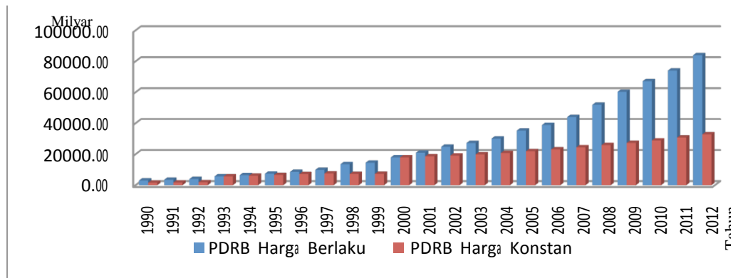
Gambar 1 Produk Domestik Regional Bruto (PDRB) atas dasar harga berlaku & konstan 2000 Periode Tahun 1990-2012
