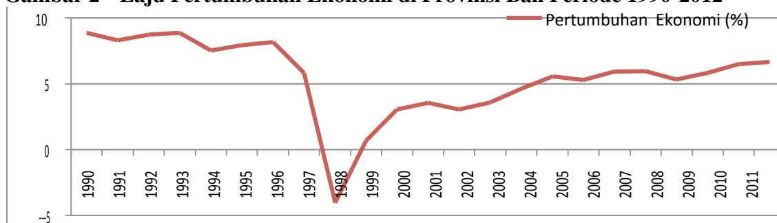
Gambar 2 Laju Pertumbuhan Ekonomi di Provinsi Bali Periode 1990-2012
