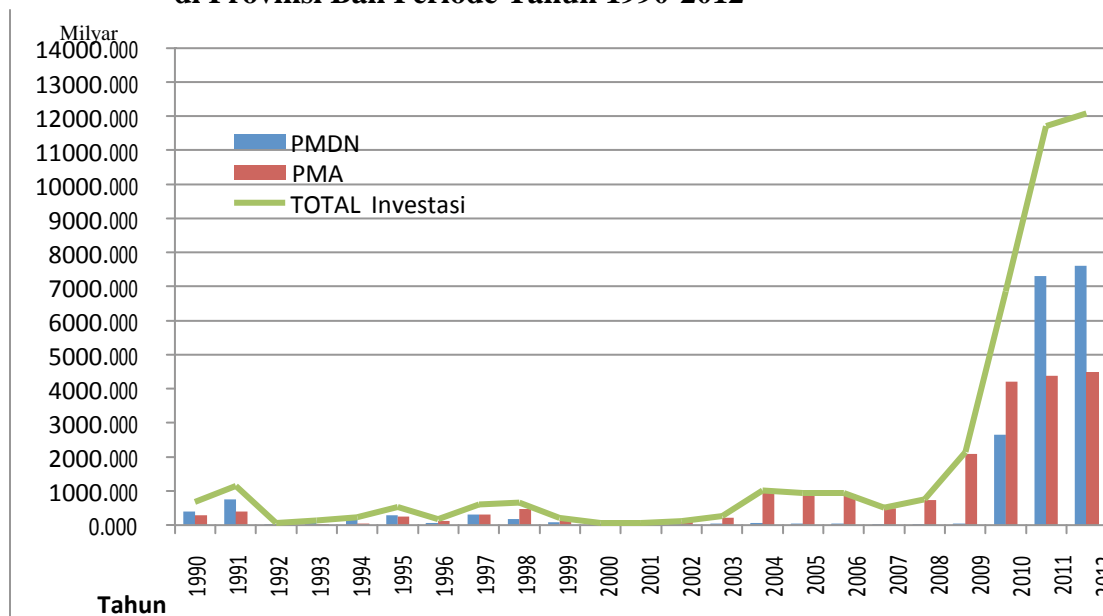
Gambar 3 Perkembangan Penanaman Modal Dalam Negeri dan Penanaman Modal Asing di Provinsi Bali Periode Tahun 1990-2012
