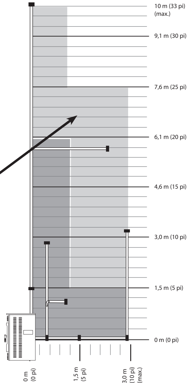
Figure 9 : Table d'évacuation et d'ajustement de tension du moteur de combustion
