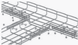
EZ T90 90-DEGREE BEND KIT, 2-PACK CBOEZT90EZ
