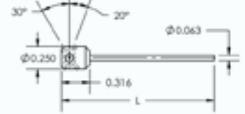
H-20/30 [TUNGSTEN HOLDER ASSEMBLY 20 & 30 DEG P/N: 002-0772]
