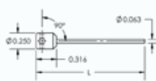
H-90 [TUNGSTEN HOLDER ASSEMBLY 90 DEG P/N: 002-0771]
