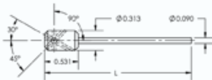
X [TUNGSTEN EXTENDER ASSEMBLY P/N: 002-0770]
