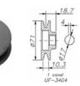
1 canal / groove
