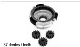
37 dentes / teeth
