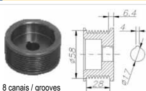
8 canais / grooves
