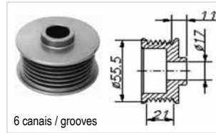
6 canais / grooves
