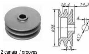
2 canais / grooves
