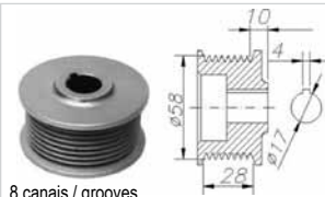
8 canais / grooves
