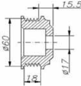
5 canais / grooves
