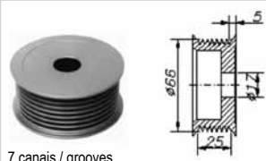
7 canais / grooves
