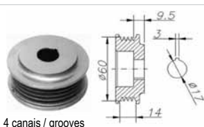
4 canais / grooves
