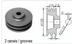
2 canais / grooves
