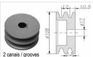
2 canais / grooves
