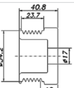
6 canal / grooves
