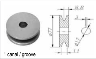
1 canal / groove
