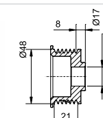
6 canais / grooves
