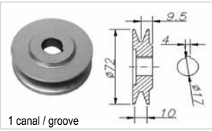
1 canal / groove
