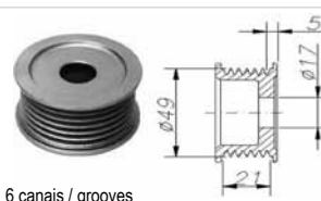
6 canais / grooves
