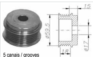
5 canais / grooves
