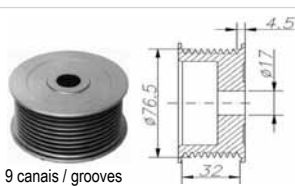
9 canais / grooves
