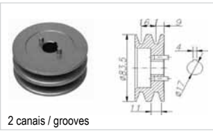
2 canais / grooves
