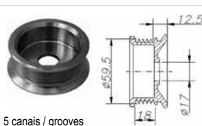
5 canais / grooves
