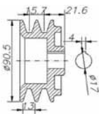
2 canais / grooves
