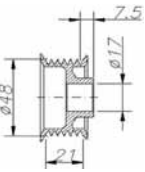
6 canais / grooves
