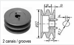
2 canais / grooves
