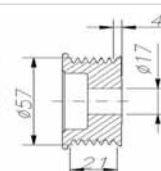
6 canais / grooves
