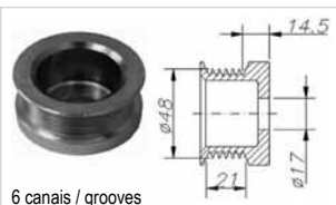
6 canais / grooves
