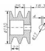
2 canais / grooves
