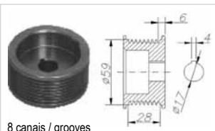
8 canais / grooves
