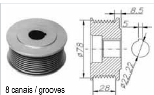
8 canais / grooves
